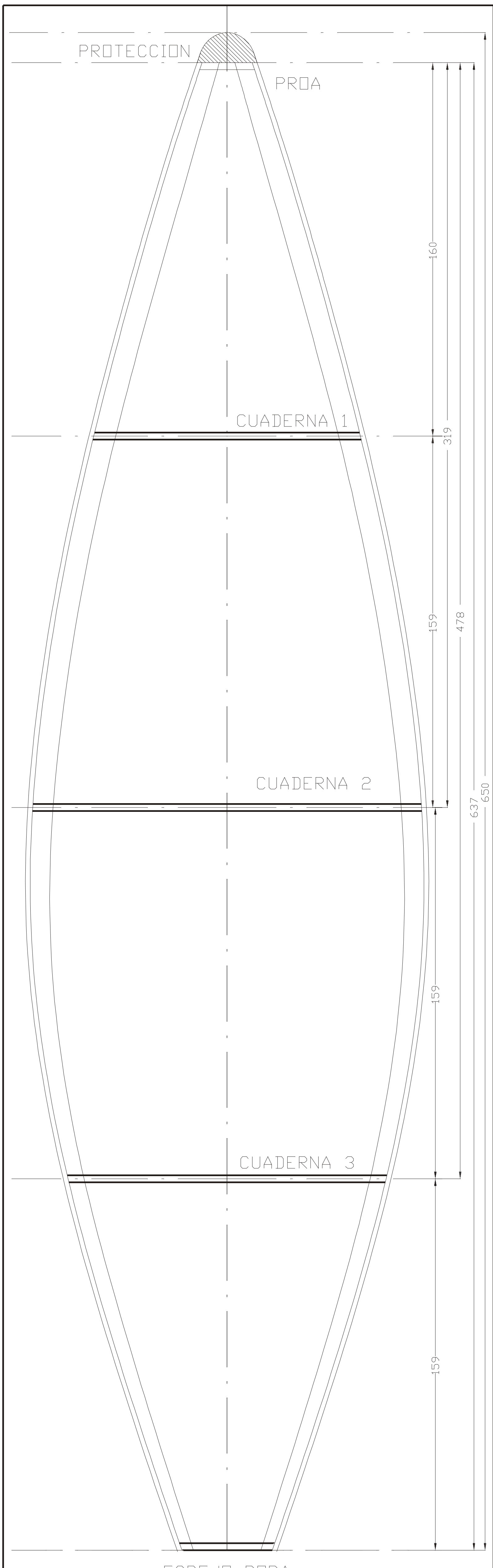
PLANO NRO.1 UBICACION DE CUADERNAS-PLANTA ESCALA 1: 1
