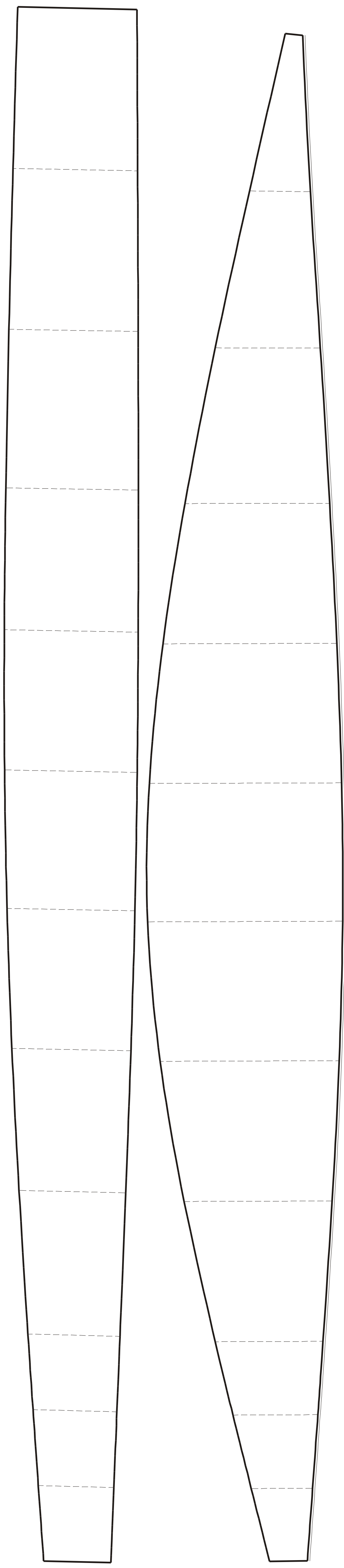
PLACAS FONDO Y LATERAL BABOR MADERA BALSA E=2mm.
