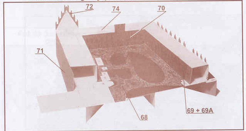
Fot.47 Konstrukcja ścian zamku średniego.
