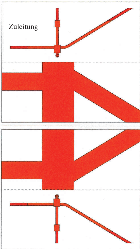
Umlaufkante Pufferbohle
