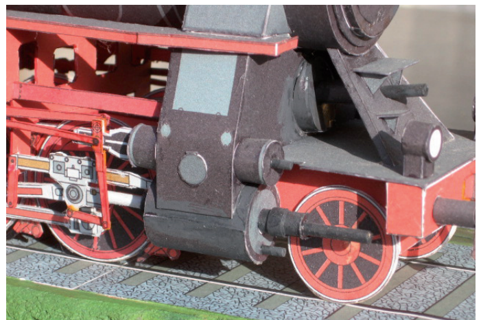
Linke Lokseite
