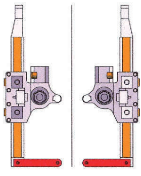
Kreuzkopf
