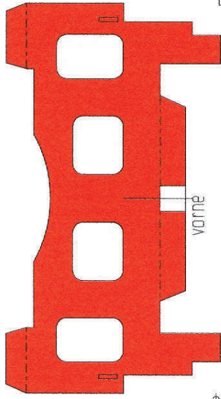
hinten Kesselstütze 2
