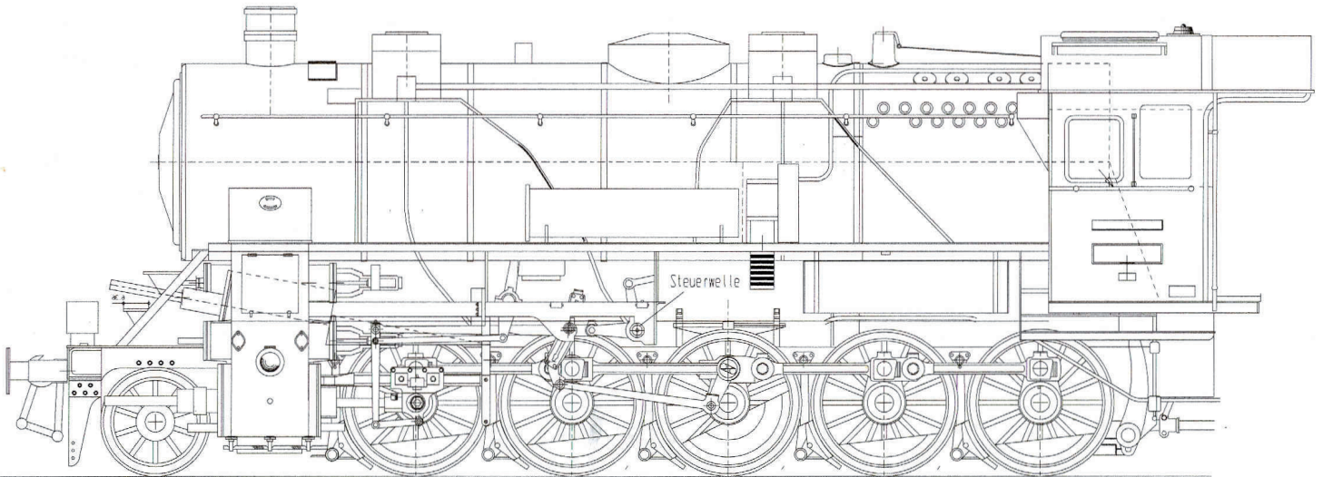
Linke Lokseite
