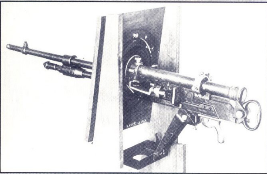
Karabin maszynowy kal.7,92 wz.25.
